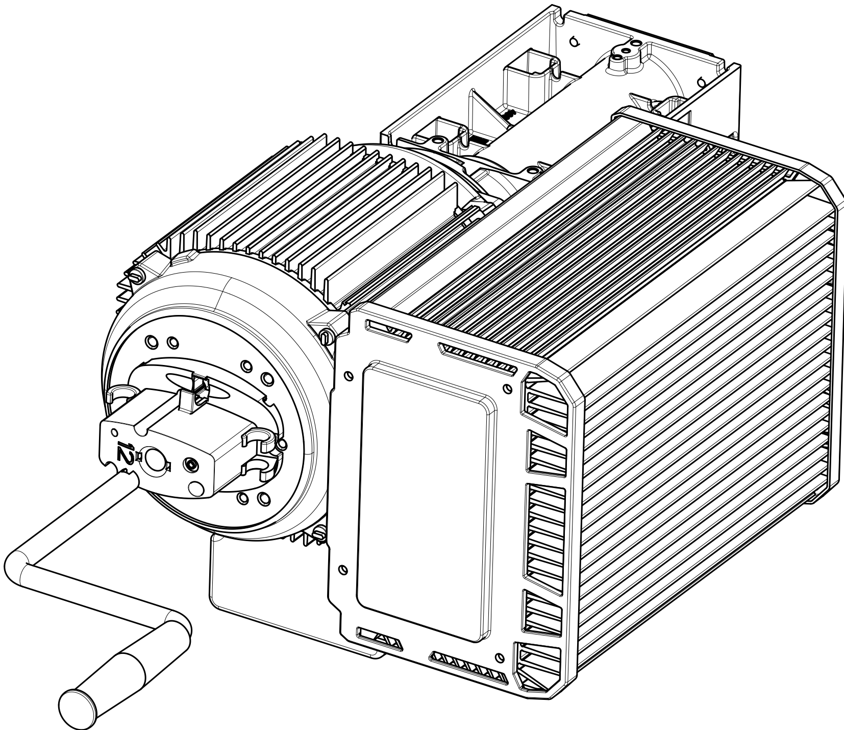
Darstellung: Einbaulage FU rechts illustration: FI on the right side
