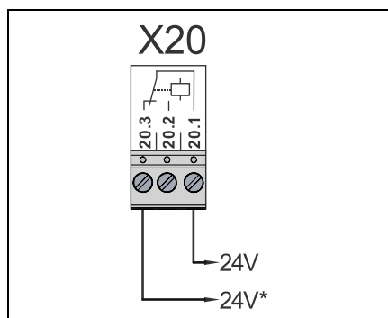
X20 : relais fonctionnel (Test de la grille lumineuse)
