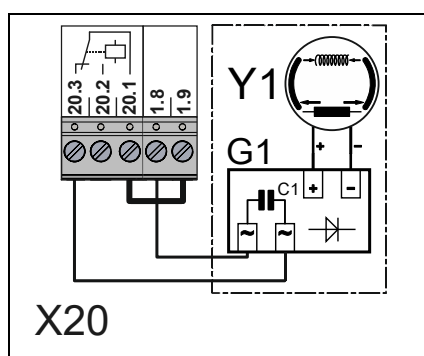
Frein magnétique G1 redresseur Y1 frein magnétique
