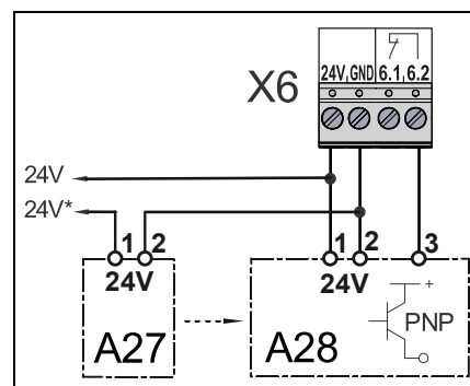
Grille lumineuse A27 : émetteur A28 : récepteur
